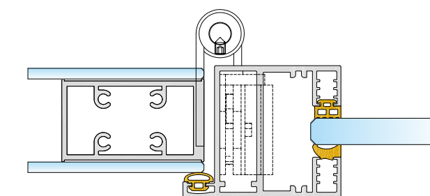
Glasdesign | Türzarge P10 | Just 3D | bis 34 dB
