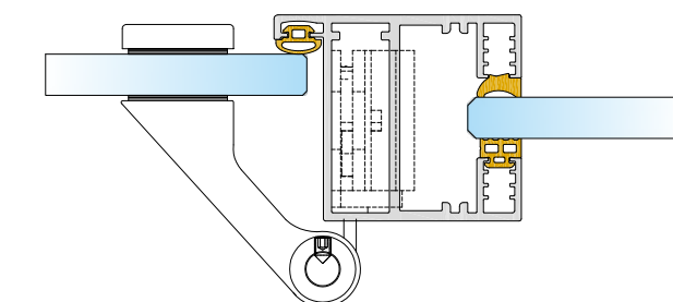
Vollglas | Türzarge P10 | Just 3D | bis 32 dB
