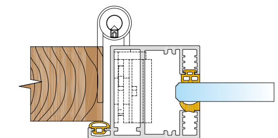
Holz | Türzarge P10 | Just 3D | bis 37 dB
