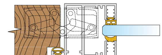
Holz | Türzarge P10 | Tectus TE 340 | bis 37 dB
